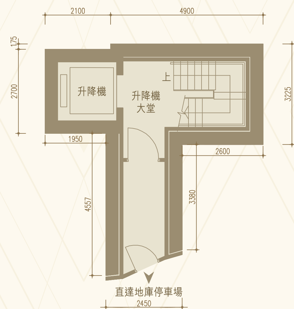
地庫平面圖
