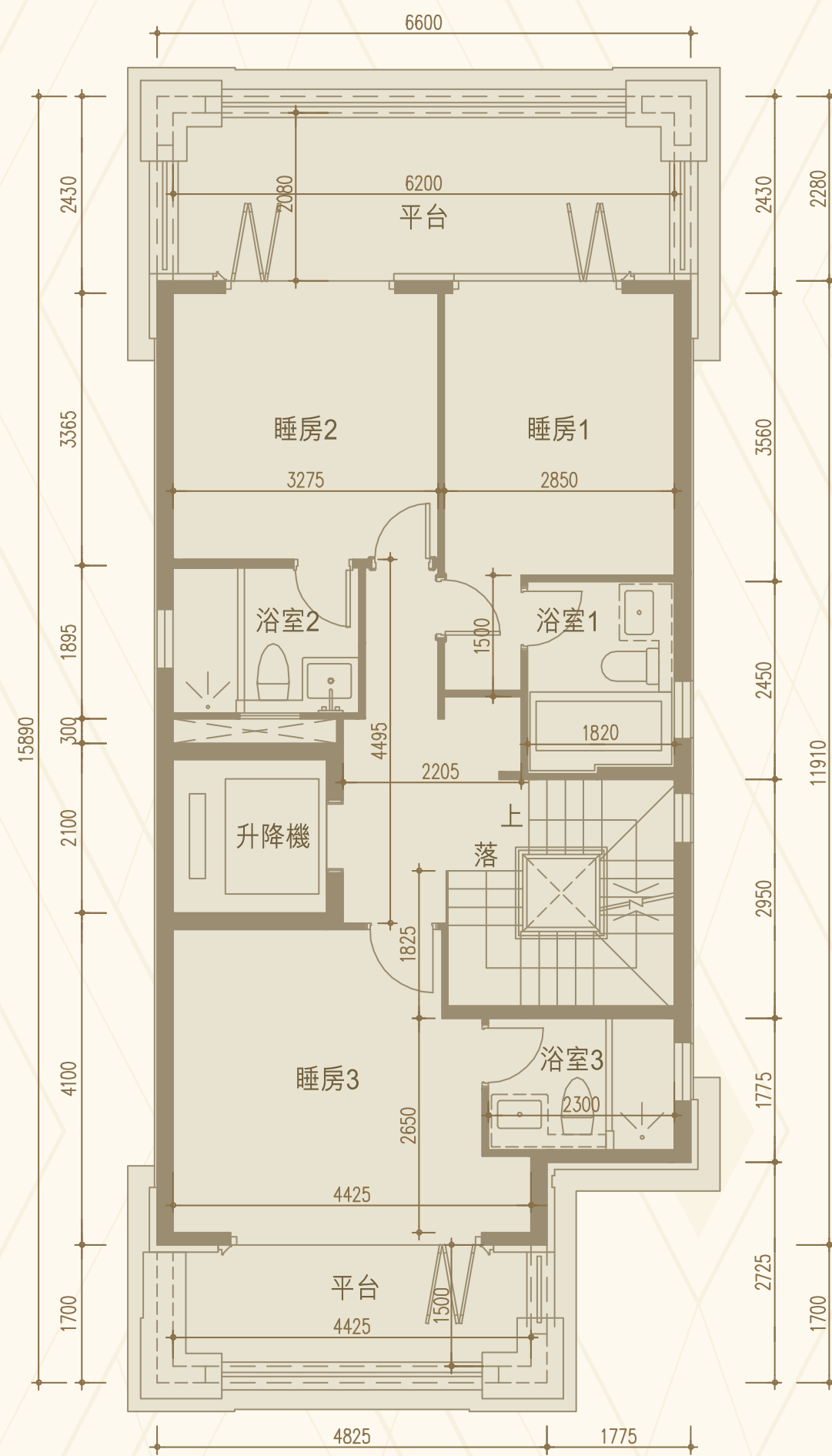
1樓平面圖
