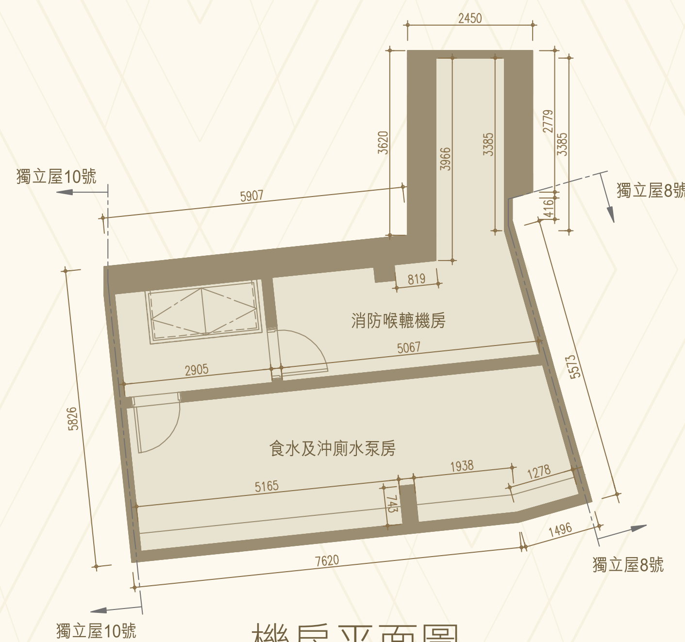
機房平面圖
