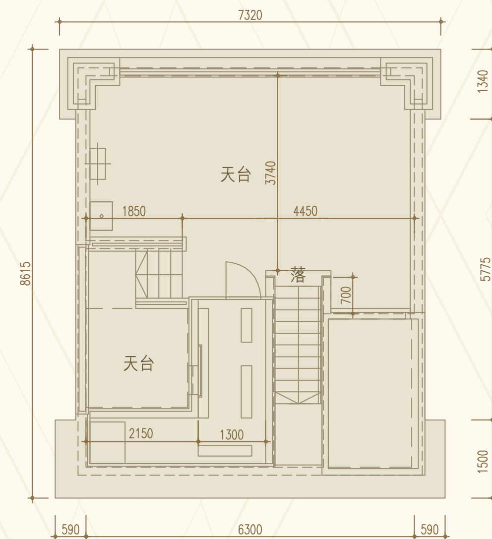
天台平面圖
